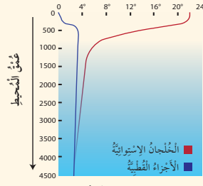
شكّل 1-1: رَسْمٌ تَمَوُّذِيٌّ لِلْمَحِيطِ الْإِسْتَوَائِيِّ يُظْهِرُ طَبَقَةَ التَّغْيِيرِ الْحَرَارِيِّ.
