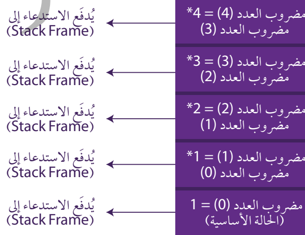
الشكل (3-4): مثال على آلية عمل الدوال الراجعة (Recursive Functions)، واستخدام (Stack Frame) في عملية التنفيذ.
