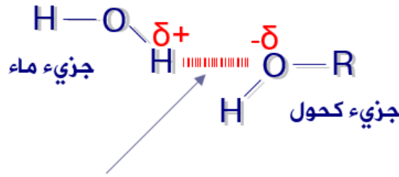
رابطه هيدروجينية
