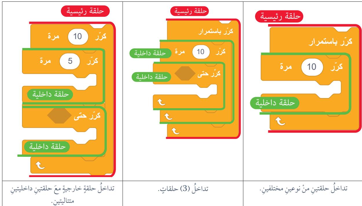
الشكل (3-7): أمثلة على أنواع الحلقات المُتداخلة.
