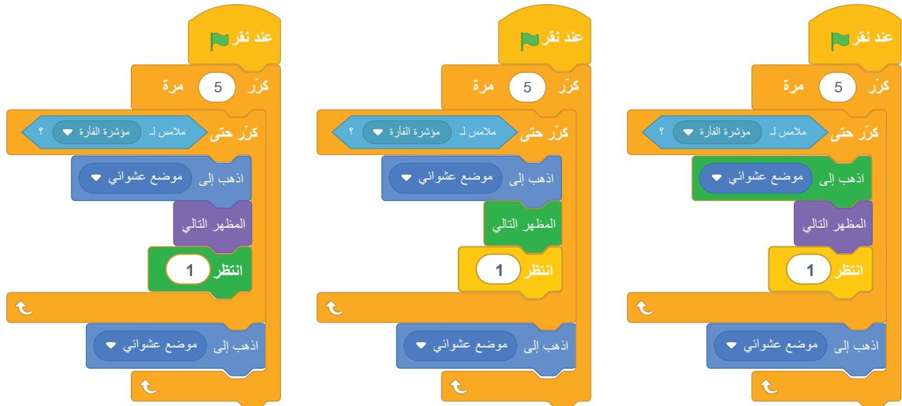
الشكل (5-3): تنفيذُ لَبَنَاتِ الحلقةِ الداخليةِ.
